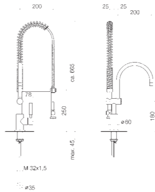
33 880 888 Professional single-lever mixer, 200 mm projection Miscelatore monocomando professionale, profondità 200 mm Mezclador monomando profesional, saliente 200 mm
