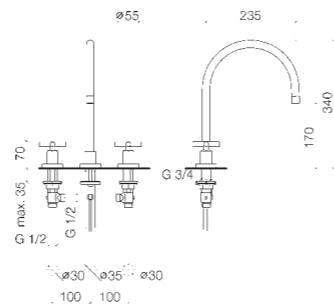
20 815 890 Three-hole mixer, 235 mm projection Batteria tre fori, profondità 235 mm Grifo mezclador con tres orificios, saliente 235 mm
