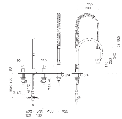
20 815 888 + 27 780 970 Three-hole mixer with profi spray set, 235 mm projection Batteria tre fori con batteria doccia professionale, profondità 235 mm Grifo mezclador con tres orificios con juego de grifo profesional tipo ducha, saliente 235 mm
