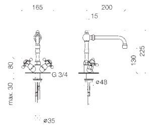
22 021 360 Single-hole mixer, 200 mm projection Batteria monoforo, profondità 200 mm Grifo mezclador con un orificio, saliente 200 mm
