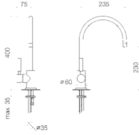
33 815 889 Single-lever mixer with lever on left, 235 mm projection Miscelatore monocomando azionamento a sinistra, profondità 235 mm Mezclador monomando con palanca a la izquierda, saliente 235 mm
