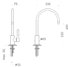
33 815 888 Single-lever mixer, 235 mm projection Miscelatore monocomando, profondità 235 mm Mezclador monomando, saliente 235 mm
