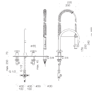
20 815 890 + 27 780 970 Three-hole mixer with profi spray set, 235 mm projection Batteria tre fori con batteria doccia professionale, profondità 235 mm Grifo mezclador con tres orificios con juego de grifo profesional tipo ducha, saliente 235 mm
