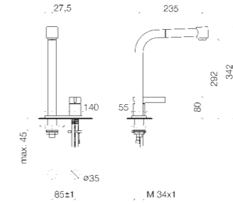
32 870 790 Two-hole mixer with extendable spray and cover plate, 235 mm projection Miscelatore monocomando a due fori con doccetta estraibile e piastra di copertura, profondità 235 mm Grifo mezclador con dos orificios con grifo estraible y cubierta, saliente 235 mm
