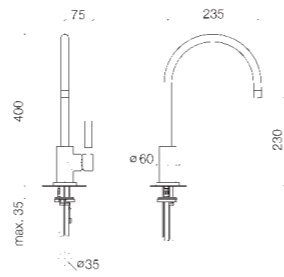
33 855 888 Single-lever mixer, 235 mm projection Miscelatore monocomando, profondità 235 mm Mezclador monomando, saliente 235 mm
