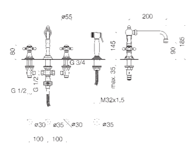
20 712 360 + 27 715 970 Three-hole mixer with rinsing spray set, 200 mm projection Batteria tre fori con gruppo doccia lavello, profondità 200 mm Grifo mezclador con tres orificios con juego de grifo para cocina, saliente 200 mm
