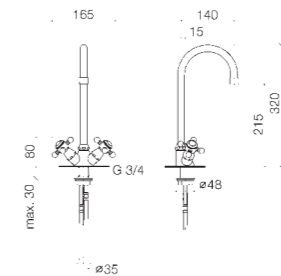
21 024 360 Single-hole mixer, 135 mm projection Batteria monoforo, profondità 135 mm Grifo mezclador con un orificio, saliente 135 mm
