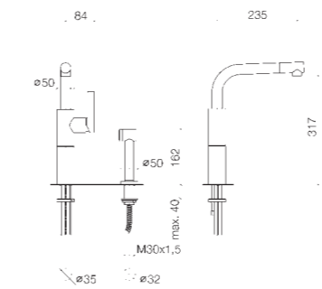
33 836 790 + 27 719 970 Single-lever mixer with base with rinsing spray set, 235 mm projection Miscelatore monocomando con zoccolo alto con gruppo doccetta livello, profondità 235 mm Mezclador monomando sobre zócalo con juego de grifo para cocina, saliente 235 mm
