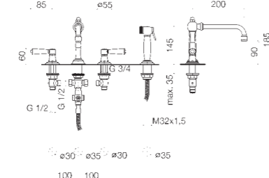
20 712 378 + 27 715 970 Three-hole mixer with rinsing spray set, 200 mm projection Batteria tre fori con gruppo doccia lavello, profondità 200 mm Grifo mezclador con tres orificios con juego de grifo para cocina, saliente 200 mm
