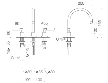
20 712 888 Three-hole mixer, 200 mm projection Batteria tre fori, profondità 200 mm Grifo mezclador con tres orificios, saliente 200 mm
